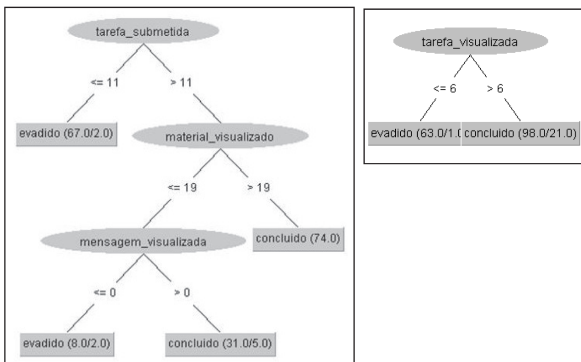
Figura 2: Árvore de decisão gerada pelo J48 para o (a) Conjunto 1 e (Conjunto 2)
